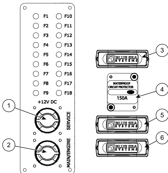
Figur 8.1 Buster Magnum Cabin hovedbrytere og sikringspanel
