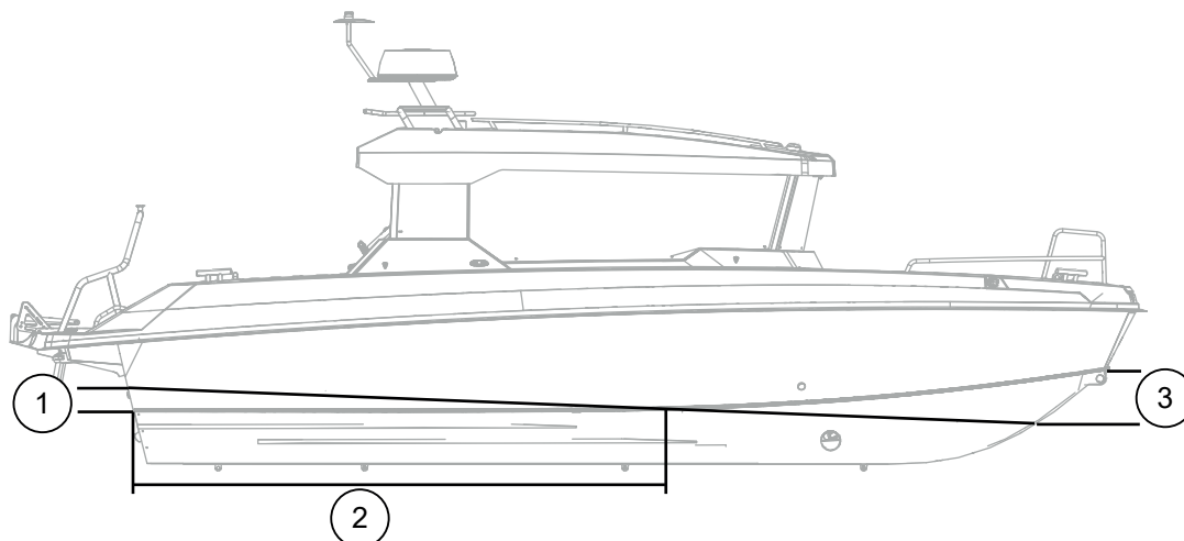
Figur 3.1 Buster Magnum Cabin bunnstoffområde
