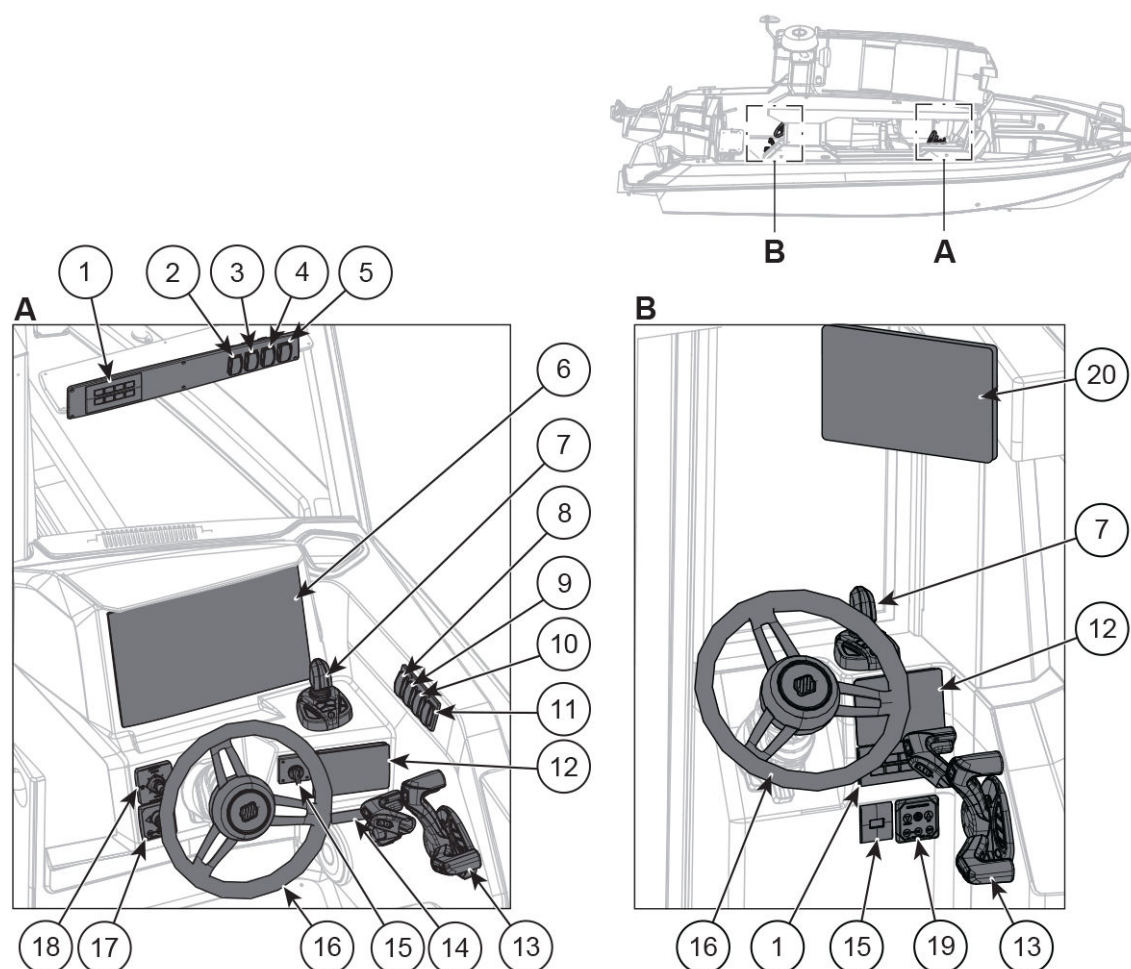
Figur 5.1 Styrestasjonskontroller i kabinen (A) og utvendige styrestasjonskontroller (B) tilgjengelig som ekstrautstyr
