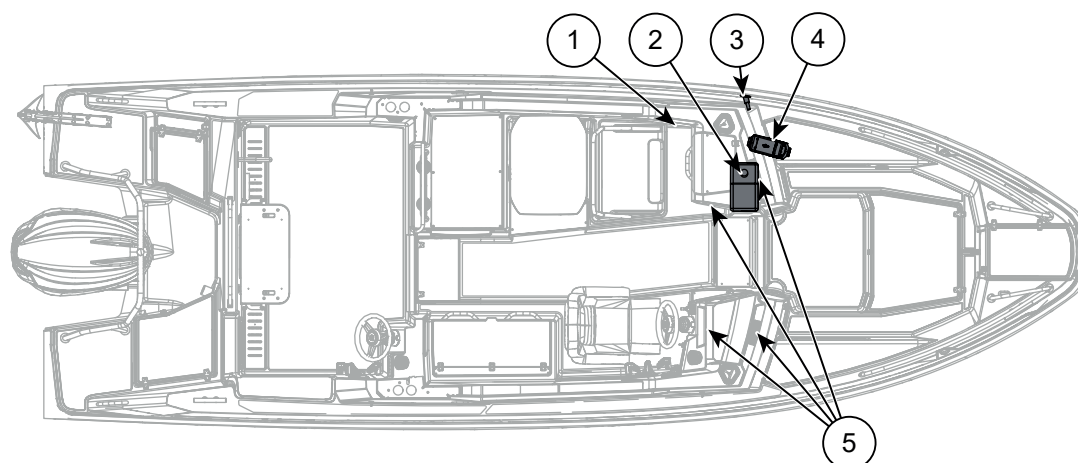
Figur 6.2 Komponenter i varmeapparat
