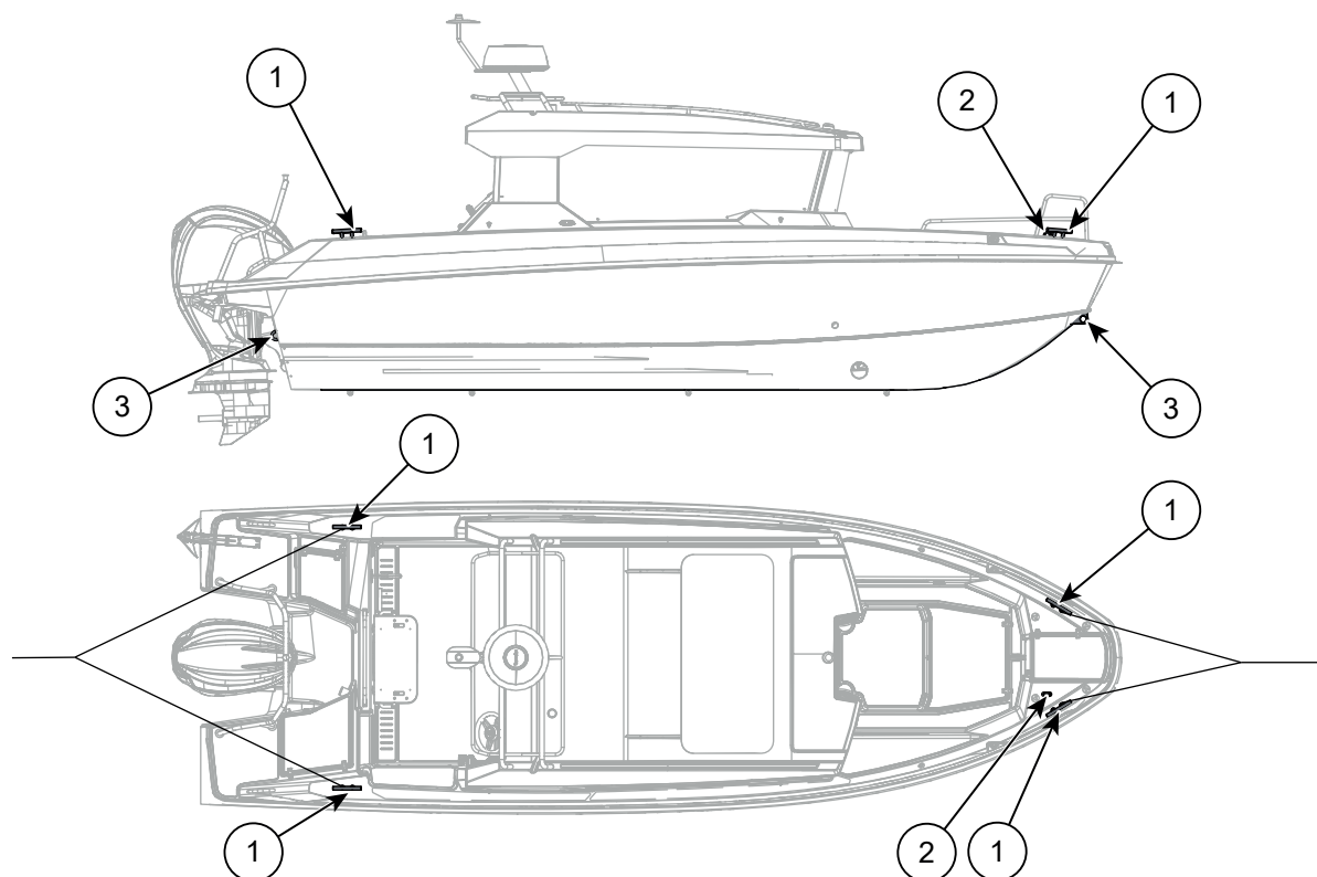
Figur 5.7 Buster Magnum Cabin fortøynings- og slepepunkter
