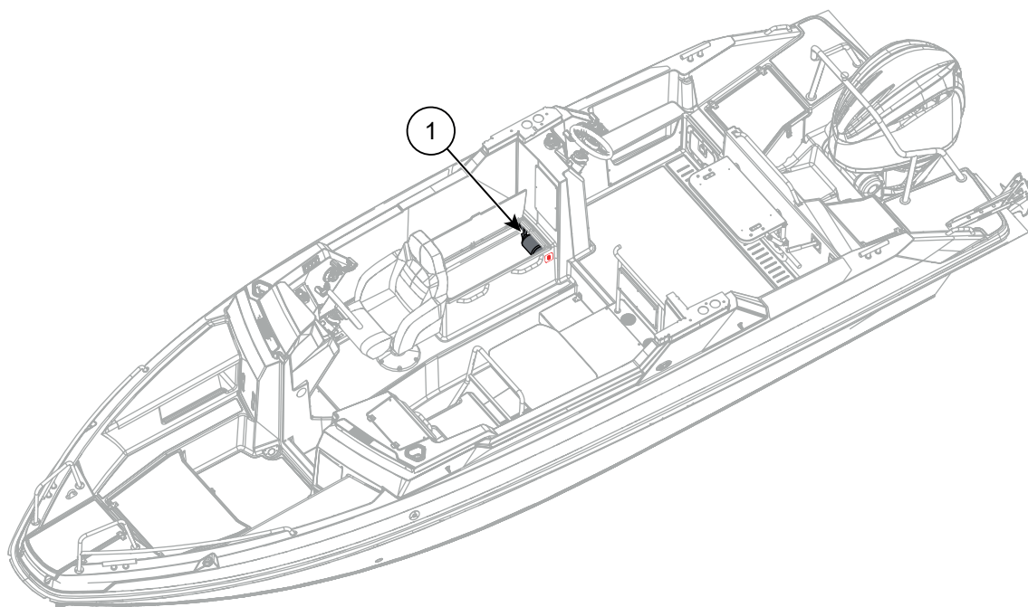
Figur 2.2 Buster Magnum Cabin plassering av brannslukningsapparat
