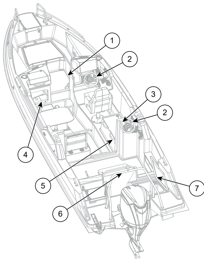
Figur 2.1 Buster Magnum Cabin sikkerhetsmerker
